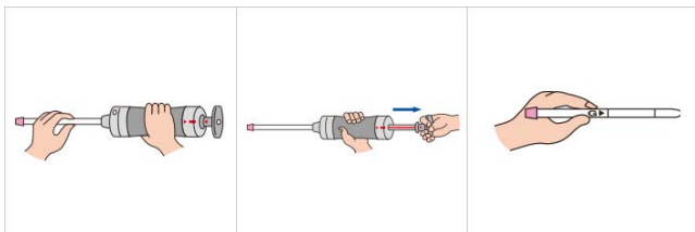
①検知管をセット ②一気にハンドルを引く ③目盛りを読む
